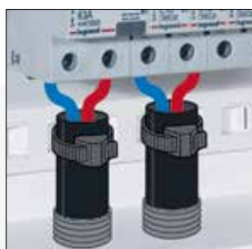
7 SUPPORTS COLLIERS Permet d'optimiser l'organisation des câbles
