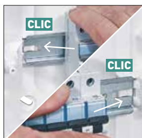
2 MONTAGE DES RAILS FACILITÉS Permet le pré-câblage en atelier. Mise en place du rail simplifiée, sans vis et sans outil.
