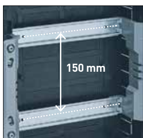
1 ENTRAXE ENTRE LES RAILS Espace de câblage optimisé pour faciliter l'accès aux bornes.
